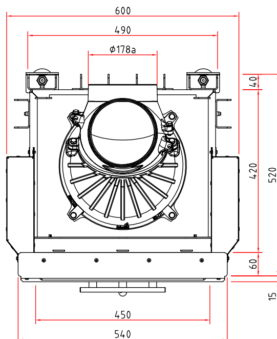
Půdorys M 1:10
